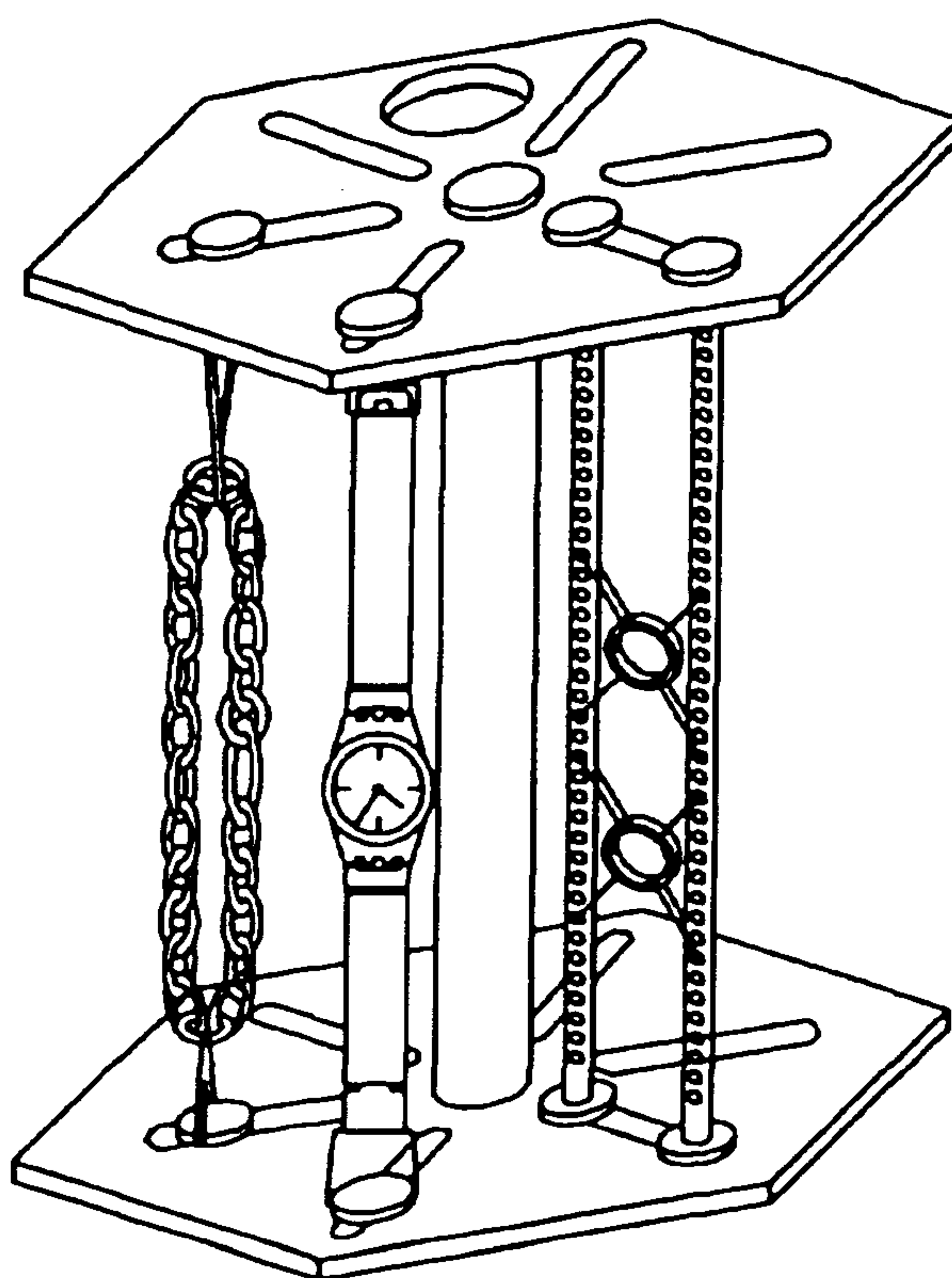
图 C.3 不同样品在支架组件上固定示例
