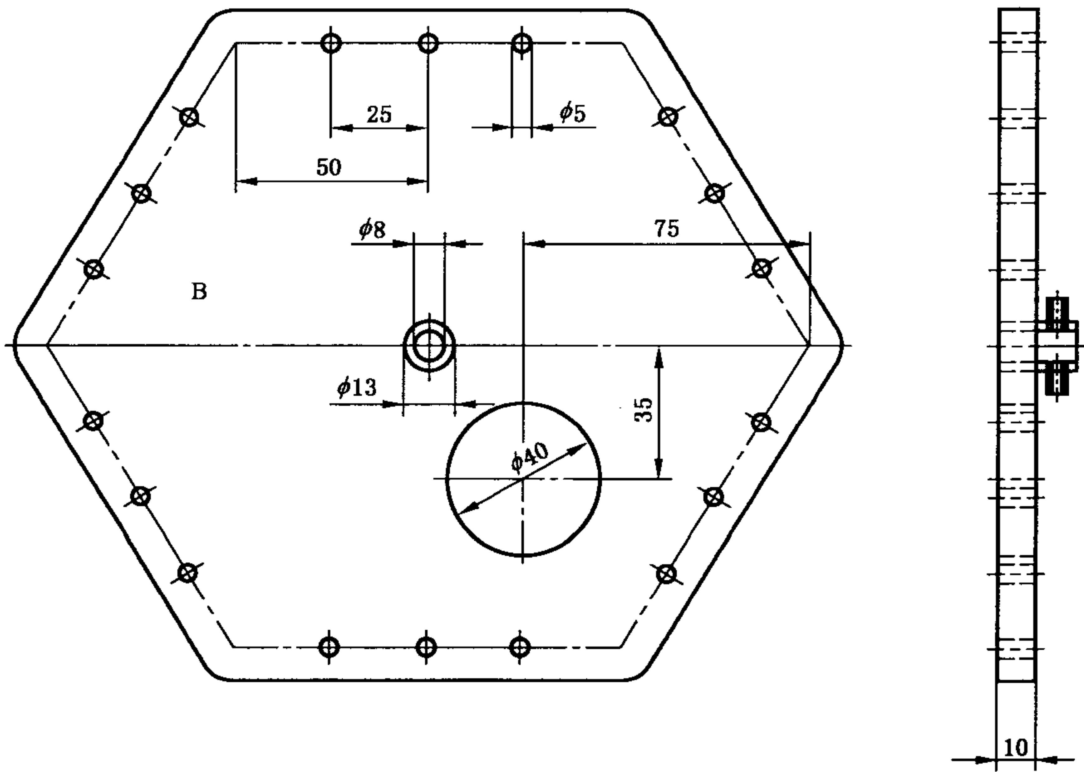
图 C.2 金属板 B 和间距螺母示意图
